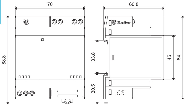
78.1C / 78.1D Schraubklemmen
