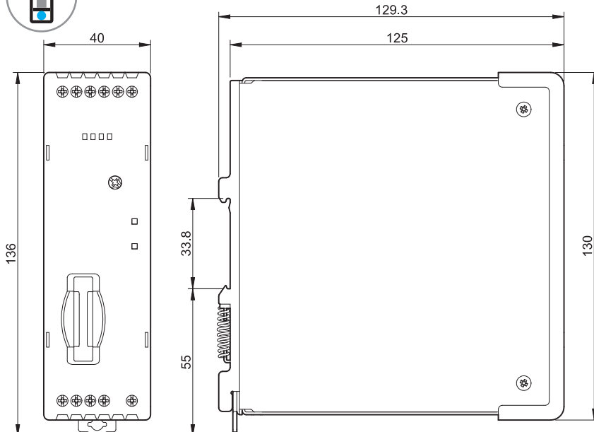
78.1C / 78.1D Schraubklemmen
