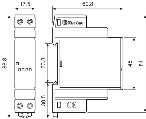
78.50 / 78.60 Schraubklemmen
