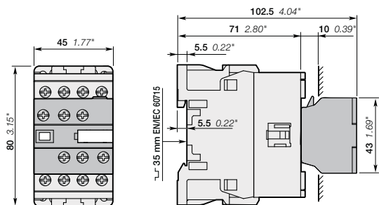
AF09, AF12, AF16 + CAT4 2-poliger Hilfskontaktblock und Spulenanschlussklemmen
