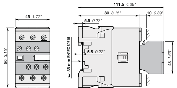
AF26, AF30, AF38 + CAT4 2-poliger Hilfskontaktblock und Spulenanschlussklemmen
