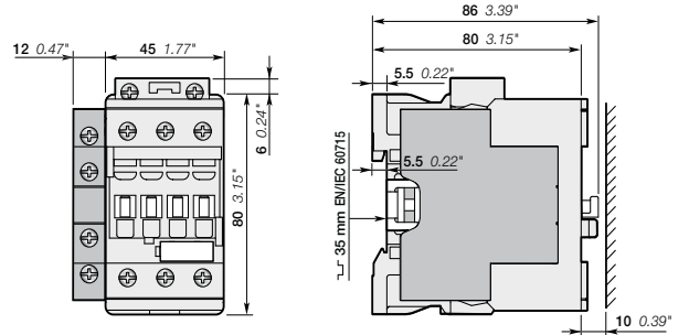
AF26, AF30, AF38 + CAL4-11 2-poliger Hilfskontaktblock
