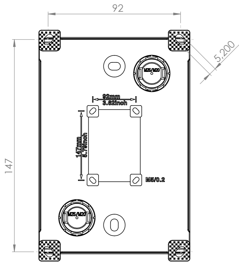
ANSICHT A
