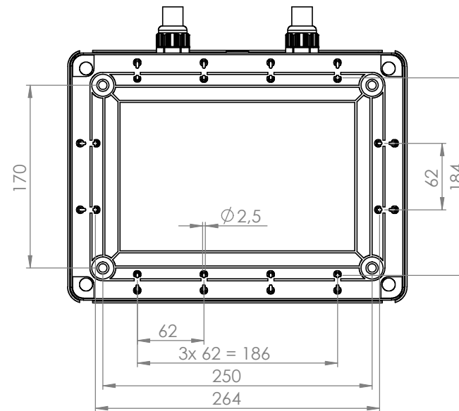
Ansicht "A"
