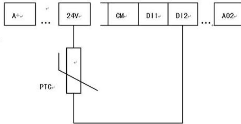
Abbildung 9-6 PTC-Überhitzungsschutz
